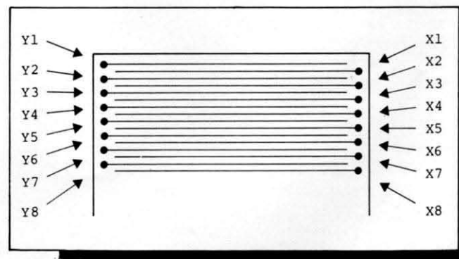
Figura 2 — Teclado visto por baixo
